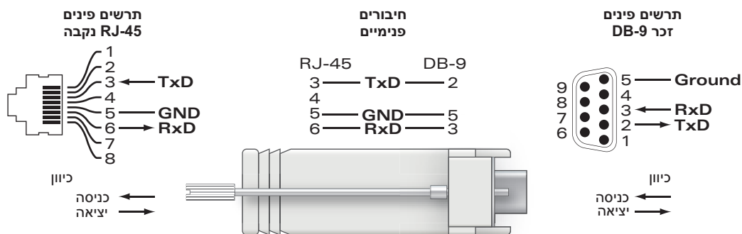
איור 5 RJ-45 מתאם המרה מודולרי (נקבה) אל DB9 (זכר)
