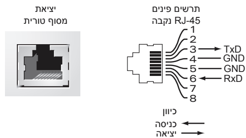
איור 4 תרשים פינים של יציאת מסוף טורית
