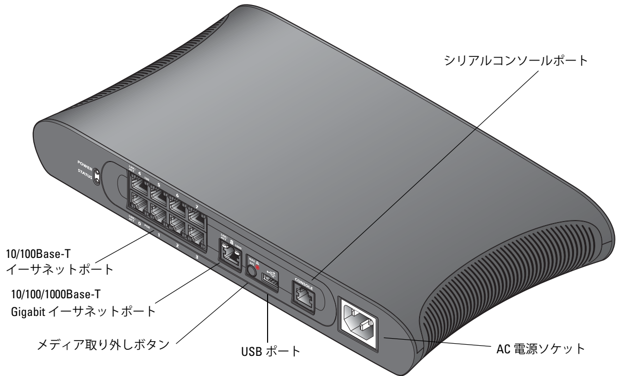
図 2 W-620 シリーズの背面
