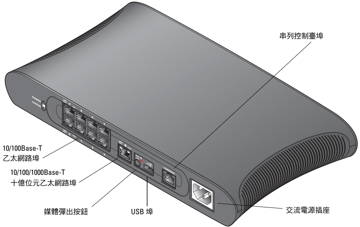
圖 2 W-620 系列系列後視圖
